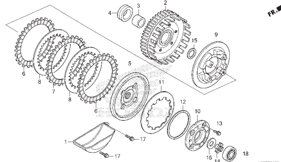
E-8 CLUTCH(FC)
