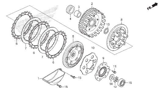
E-8-1 CLUTCH(EX)
