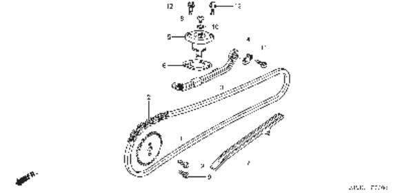
E-3 CAM CHAIN/TENSIONER
