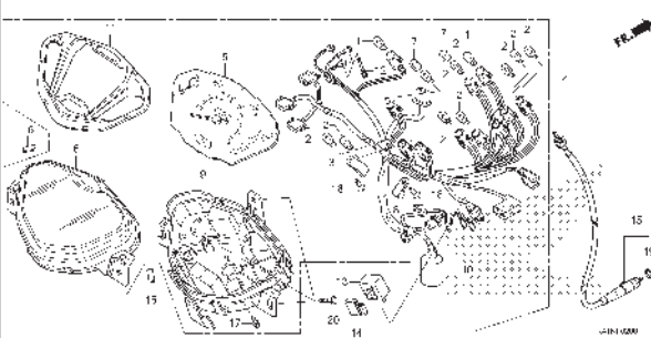
F-2 METER
