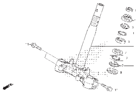
F-10 STEERING STEM
