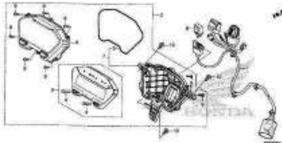
F-2-1 METER (ACB125CBFK/CBTK)
