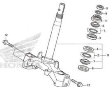
F-10 STEERING STEM
