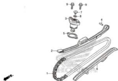
E-5 CAM CHAIN/TENSIONER
