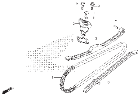
E-5 CAM CHAIN/TENSIONER
