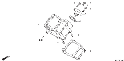
E-5 CYLINDER/TENSIONER
