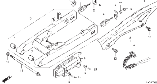
F-23 SWINGARM
