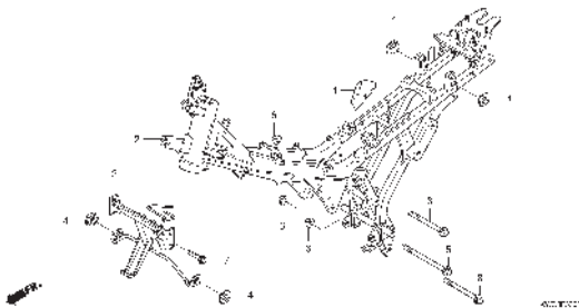
F-30 FRAME BODY
