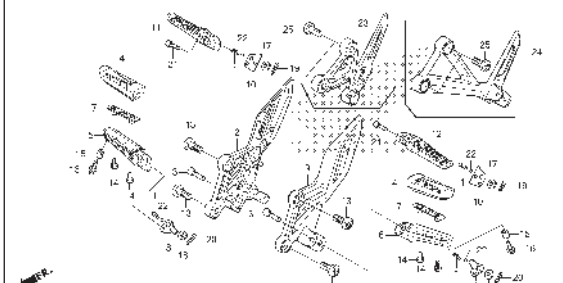
F-30 STEP
