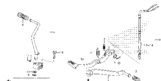
F-29 PEDAL
