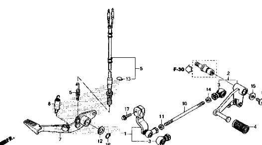
F-29 PEDAL
