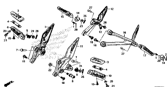
F-30 STEP
